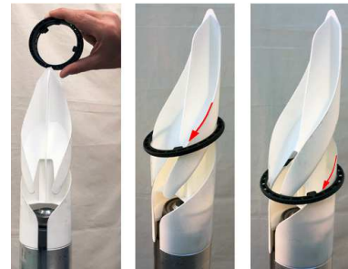
リングを回転軸に装着すれば、手で調整する必要はなく、それぞれが正確に溝へ落ちていくくみ
