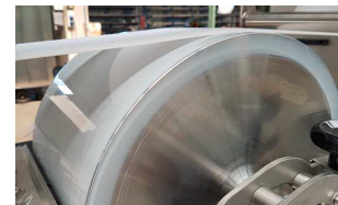
MFR FCの心臓部である片面コーティング用のリックロールユニット
